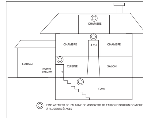
Fig 2. Schéma de l'emplacement du détecteur
